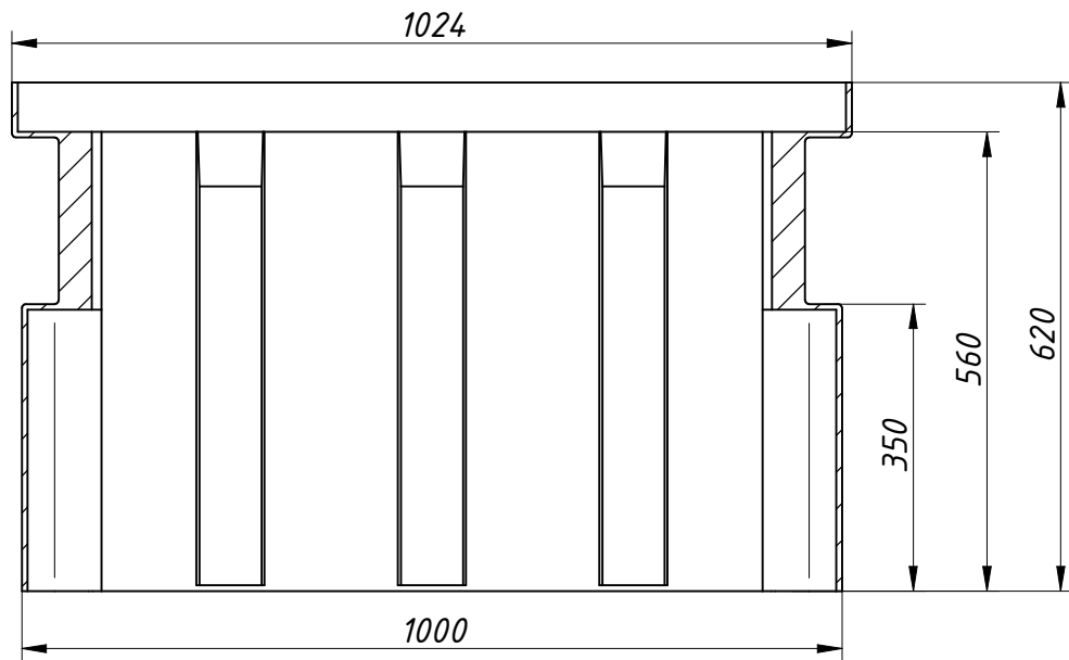
METSZET A-A
